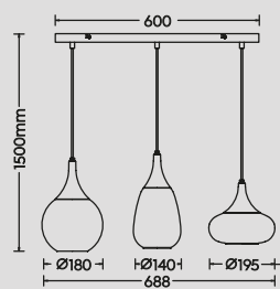
Pendelleuchte · Pendant excl. 3 x E14 max. 40 W 317000313 NEW 317000332
