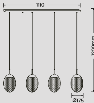
Pendelleuchte · Pendant excl. 4 x E27 max. 25 W 364200417
