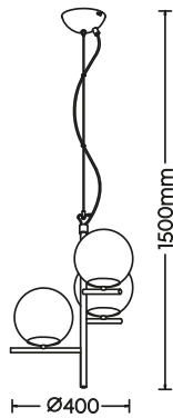
Pendelleuchte · Pendant excl. 3 x E14 max. 28 W 302000308
