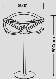
Tischleuchte · Table lamp incl. SMD-LED 26 W / 2.500 Lumen 3.000 Kelvin 521210107 521210108
