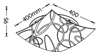
Deckenleuchte · Ceiling lamp excl. 2 x E27 max. 40 W 604400201
