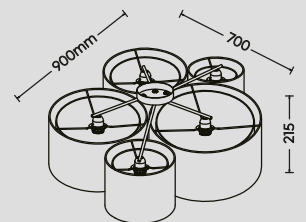
Deckenleuchte · Ceiling lamp excl. 5 x E27 max. 40 W 611400532
