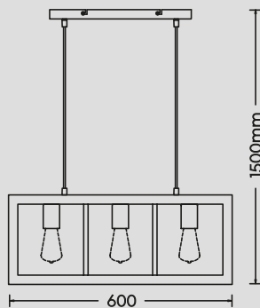
Pendelleuchte · Pendant excl. 3 x E27 max. 10 W 313800332
