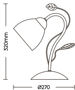
Tischleuchte · Table lamp excl. 1 x E14 max. 40 W 500700128
