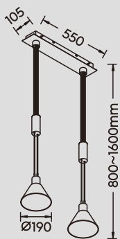
Pendelleuchte · Pendant excl. 2 x E27 max. 40 W 319500207 319500232
