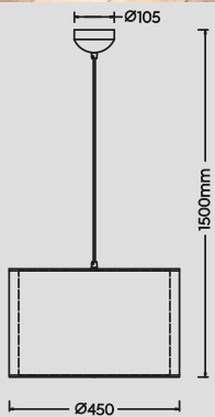
Pendelleuchte · Pendant excl. 1 x E27 max. 40 W 311400132
