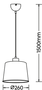
Pendelleuchte · Pendant excl. 1 x E27 max. 60 W 312700132
