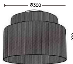
Deckenleuchte · Ceiling lamp excl. 4 x E27 max. 10 W 666800136
